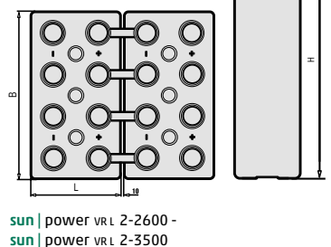
Abb. F Baureihe OPzV
